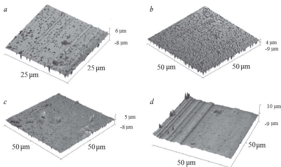
Рис. 2. Топография поверхности исходных ТМ (а), после плазменной модификации (b), после стерилизации (1 кГр) исходных (с) и плазменно модифицированных ТМ (d)
