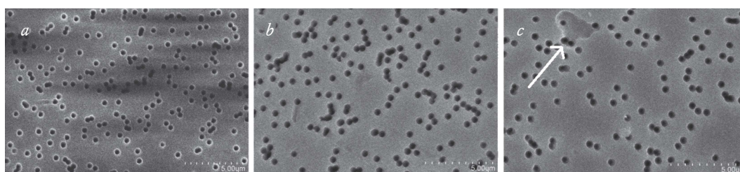
Рис. 1. Электронно-микроскопическое изображение поверхности исходной ТМ (а), ТМ после плазменной модификации (b) и после стерилизации дозой 1 кГр (с)
